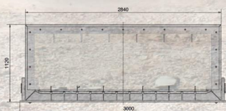
Module dimensions
